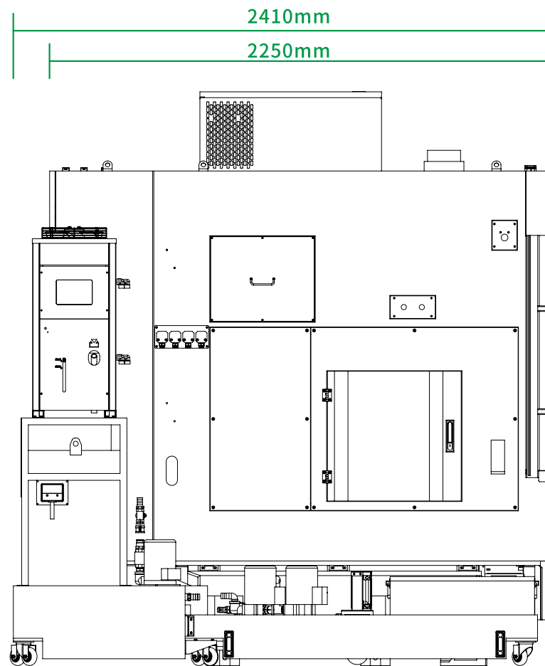
侧视图
