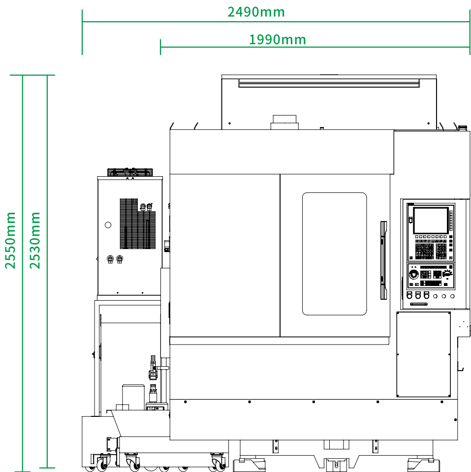
前视图
